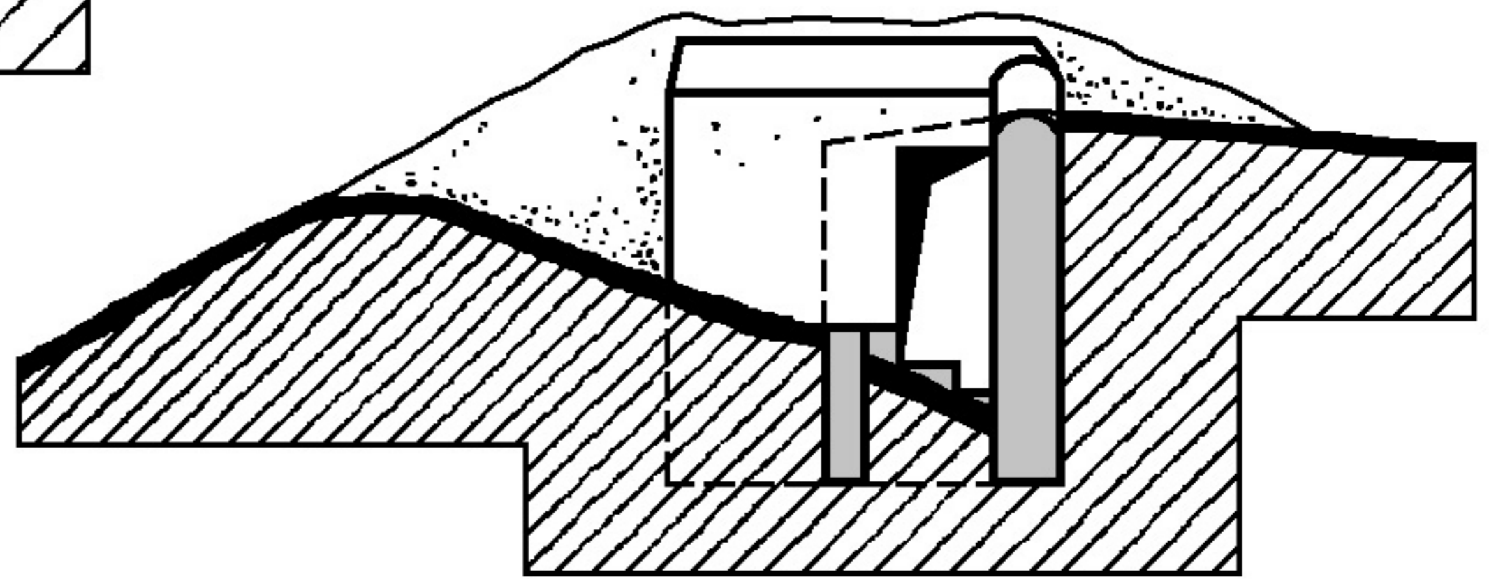
ŘEZ B-B'
