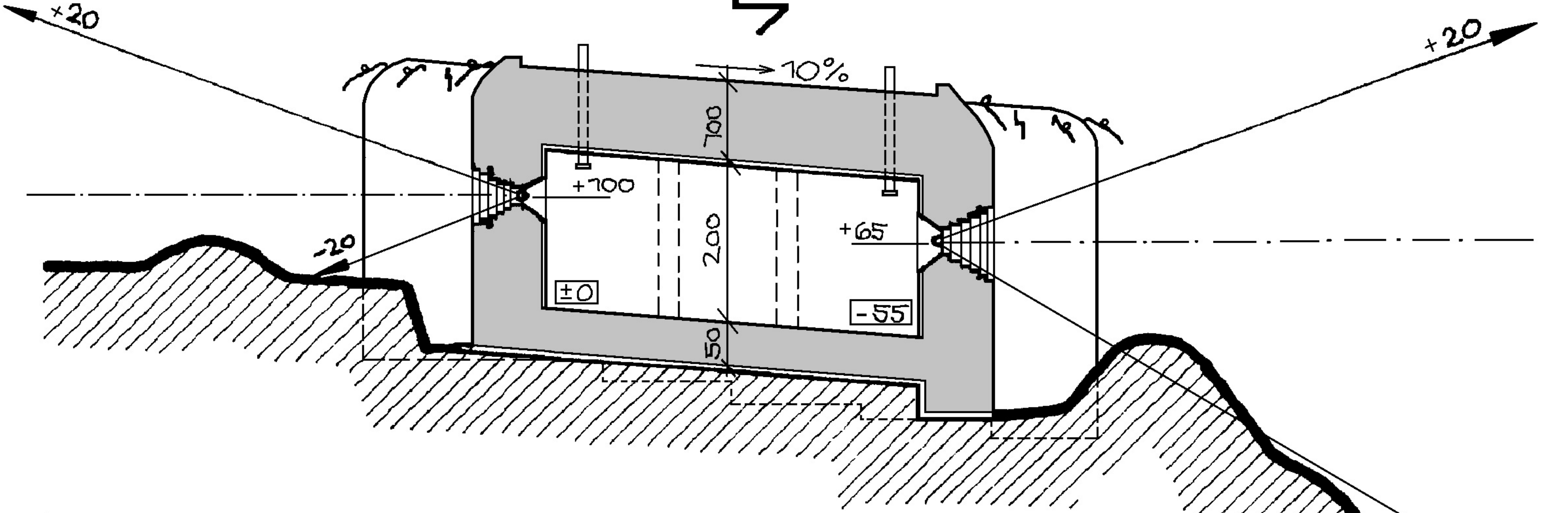
REZ B-B'
