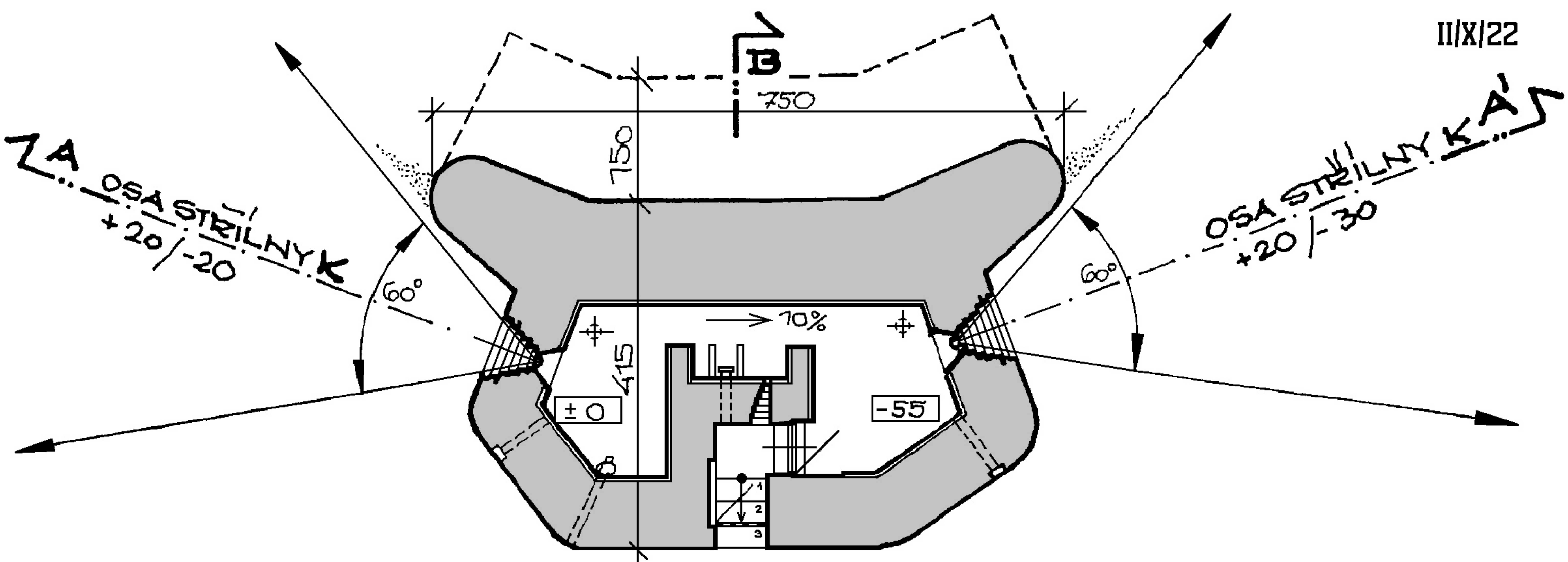
REZ A-A'
