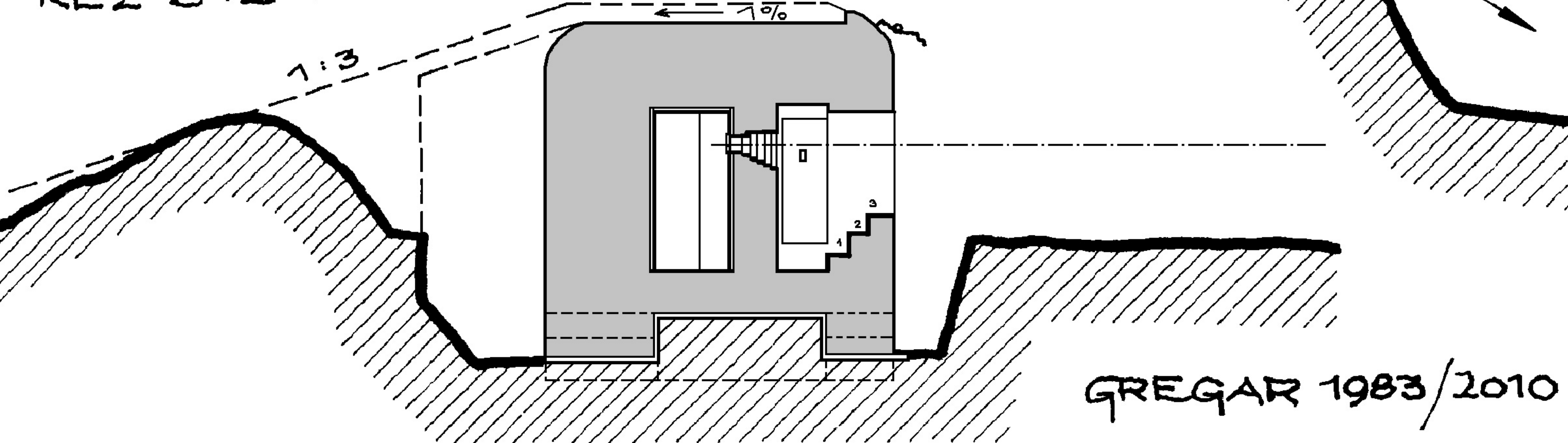
REZ B-B'
