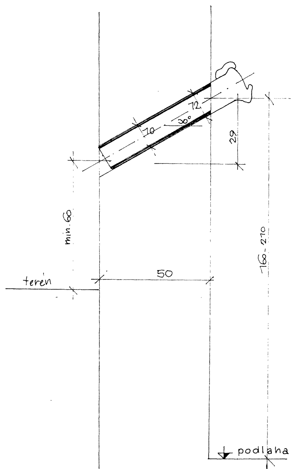
DETAIL SKLUZU 1:10
